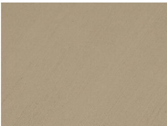
Pumice
