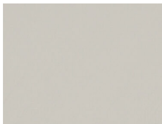
Gypsum
