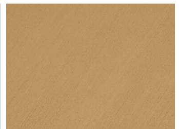
Laterite
